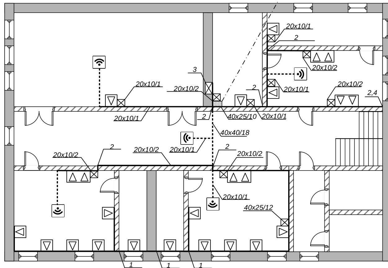
Первый этаж
